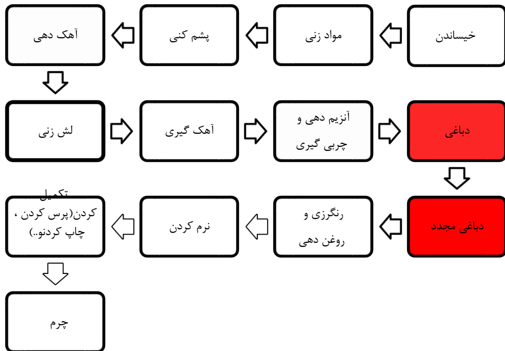
شکل ۱۵. فرایند تولید چرم طبیعی
