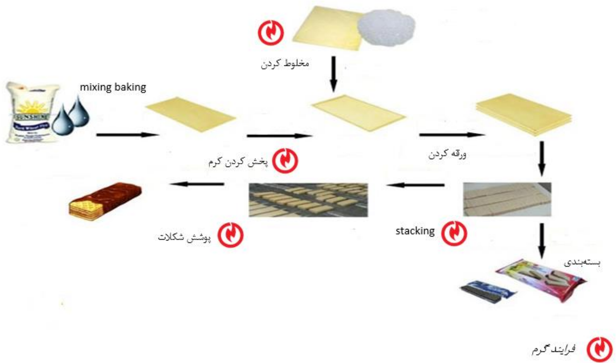
شکل ۳۱. شماتیک کلی از فرایند تولید ویفر
