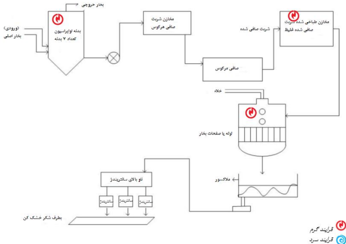
شکل ۳۴. نمای شماتیک فرآیند تغلیظ در صنعت قند و شکر
