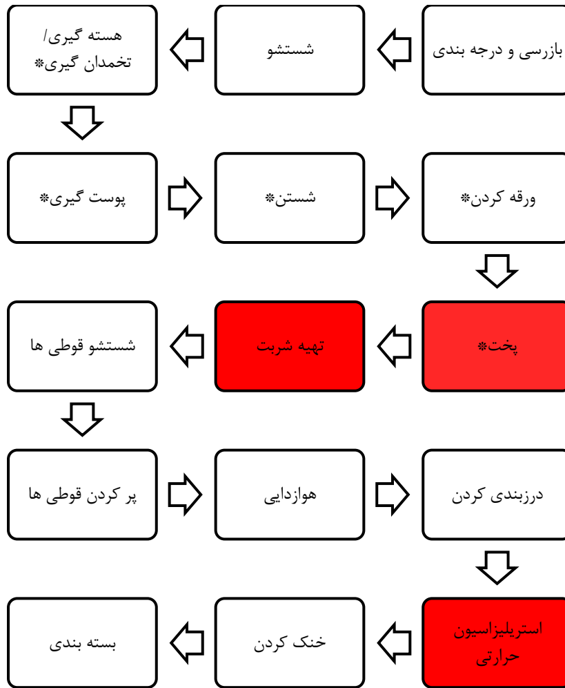
شکل ۱۷. فلوچارت فرآیند تولید در صنعت تولید کمپوت میوه *لزوماً برای همه میوه‌ها و سبزیجات اتفاق نمی‌افتد.
