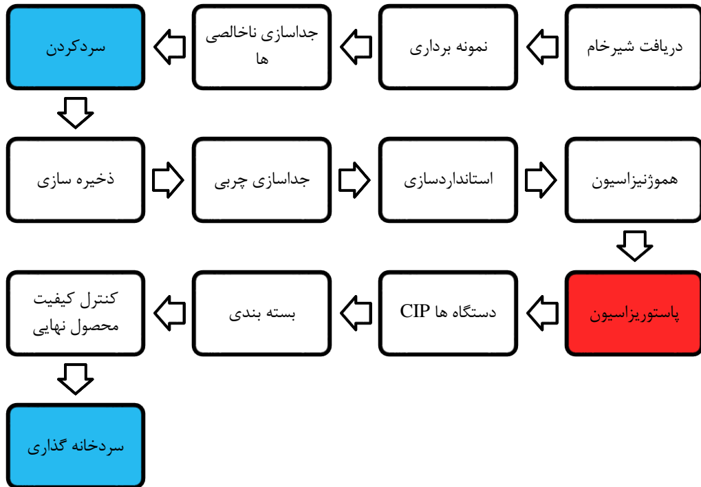
شکل ۳۵. فلوجارت پاستوریزاسیون شیر
