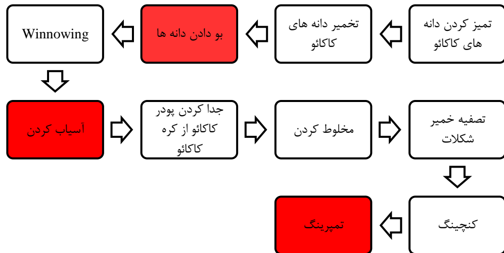
شکل ۱۹. فلوجارت فرایند تولید در صنعت شکلات و کاکائو
