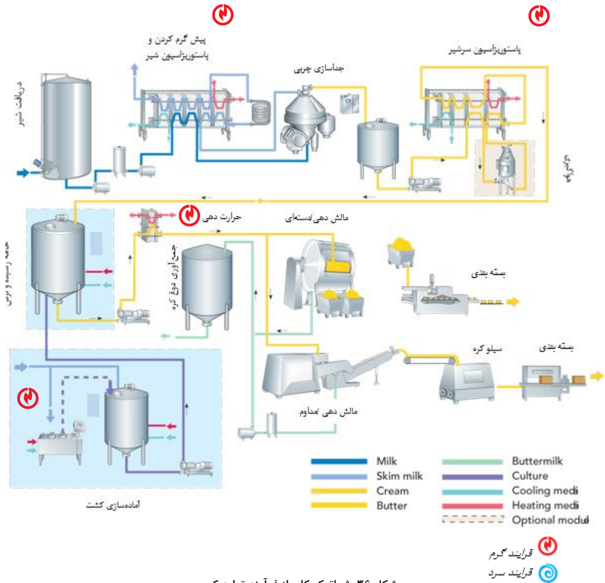
شکل ۳۶. شماتیک کلی از فرآیند تولید کره
