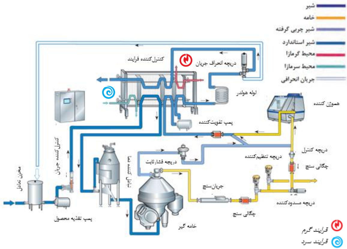
شکل ۳۴. شماتیک کلی از فرآیند پاستوریزاسیون شیر
