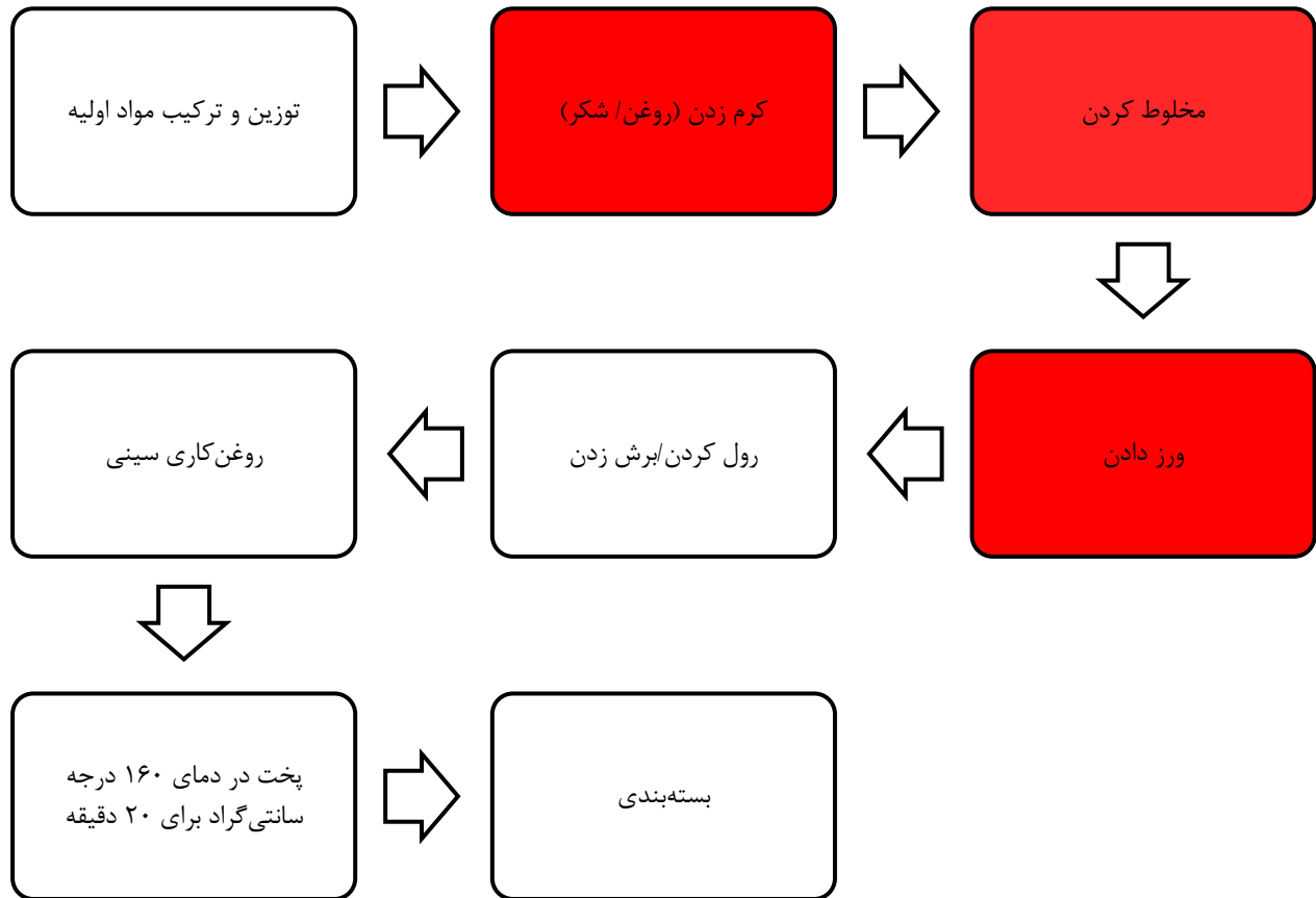
شکل ۳۲. فلوچارت تولید در صنعت ویفر
