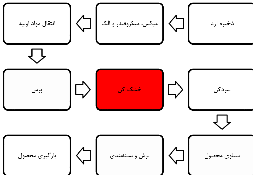
شکل ۲۹. فرآیند تولید ماکارونی
