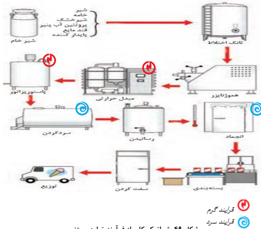
شکل ۴۹. شماتیک کلی از فرآیند تولید بستنی
