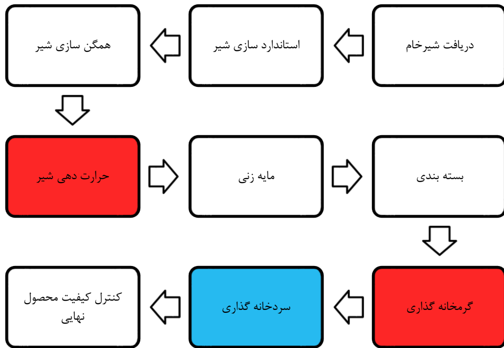
شکل ۴۰. فلوجارت تولید ماست هم نزده
