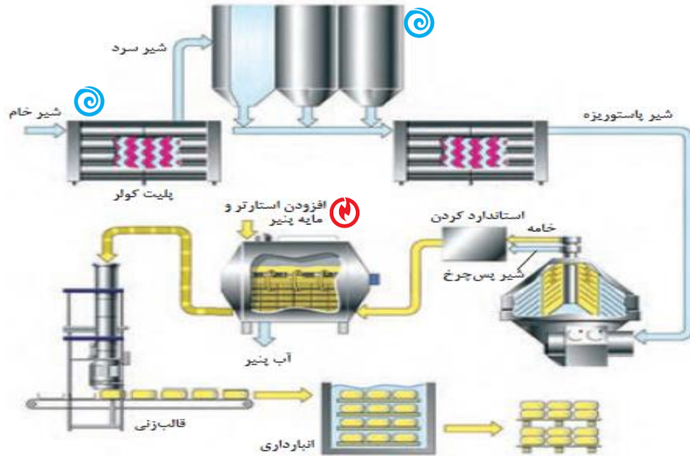
شکل ۴۷. شماتیک کلی از فرآیند تولید پنیر
