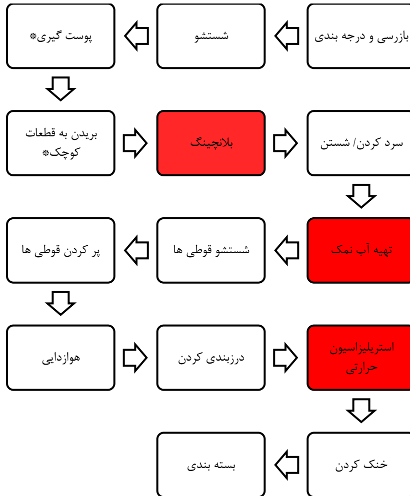
شکل ۱۸. فلوجارت فرآیند تولید در صنعت تولید کنسرو سبزیجات
