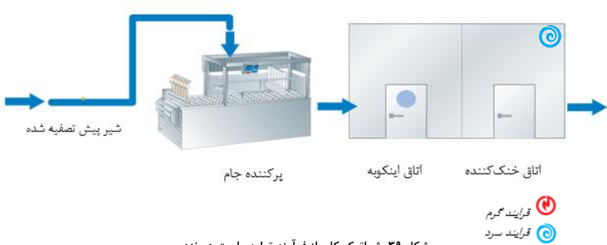
شکل ۳۹. شماتیک کلی از فرآیند تولید ماست هم نزده
