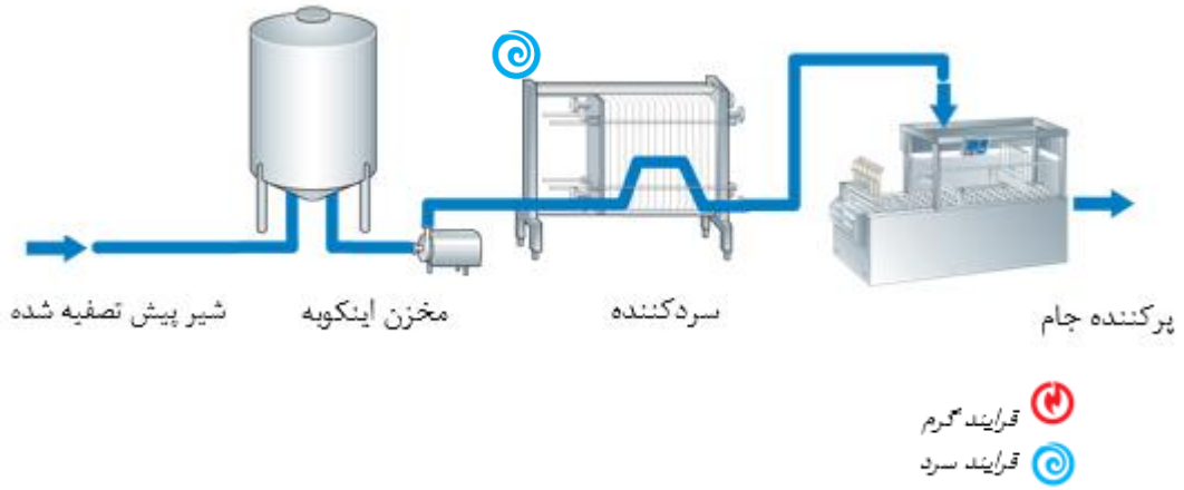
شکل ۴۱. شماتیک کلی از فرآیند تولید ماست هم زده
