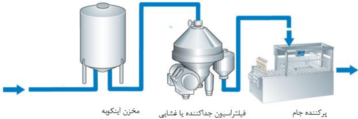
شکل ۴۵. شماتیک کلی از فرآیند تولید کشک
